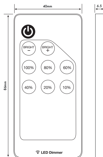
Mini RF Remote Controller SCD107W
